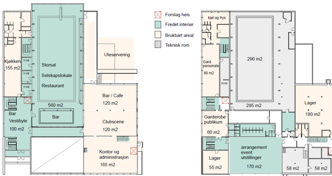
Figur 7: Skisse som viser mulig planløsning for konsept 2.
