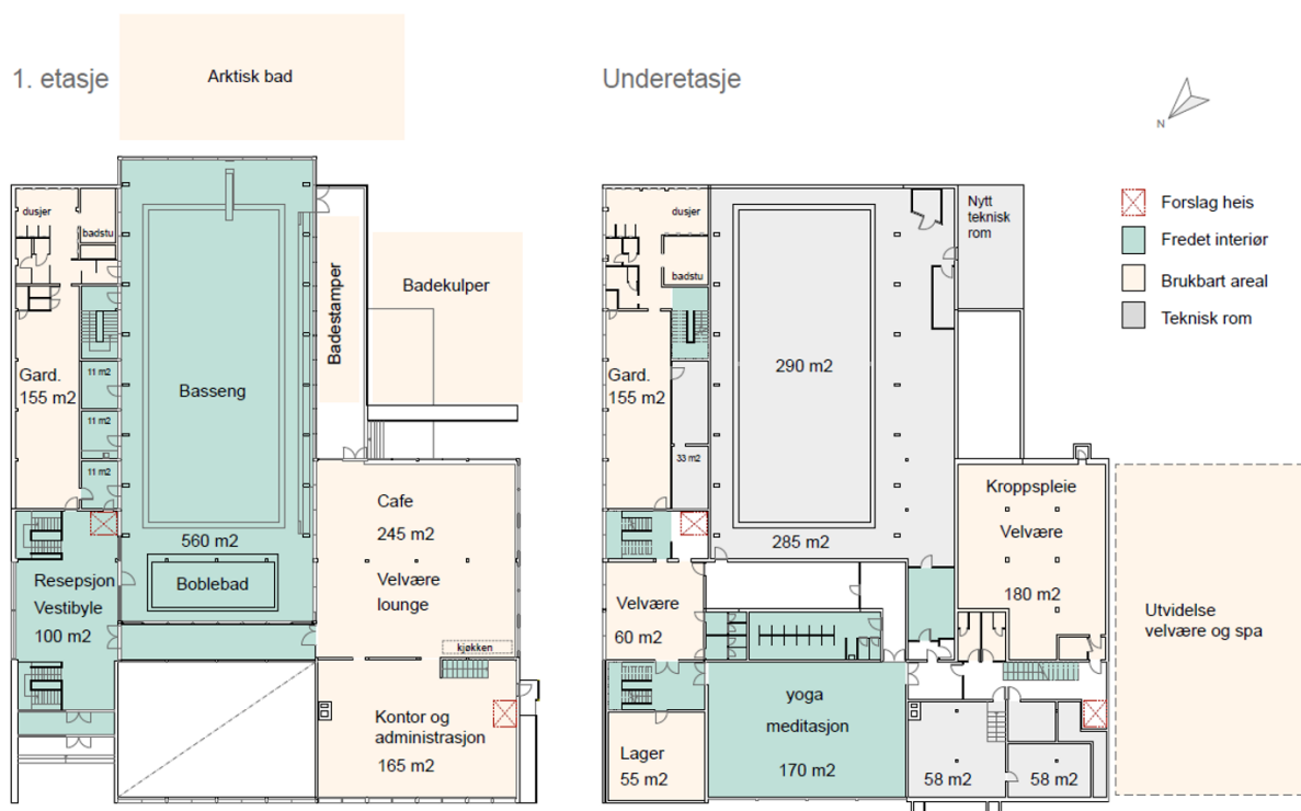
Figur 9: Skisse som viser mulig planløsning for konsept 4.
